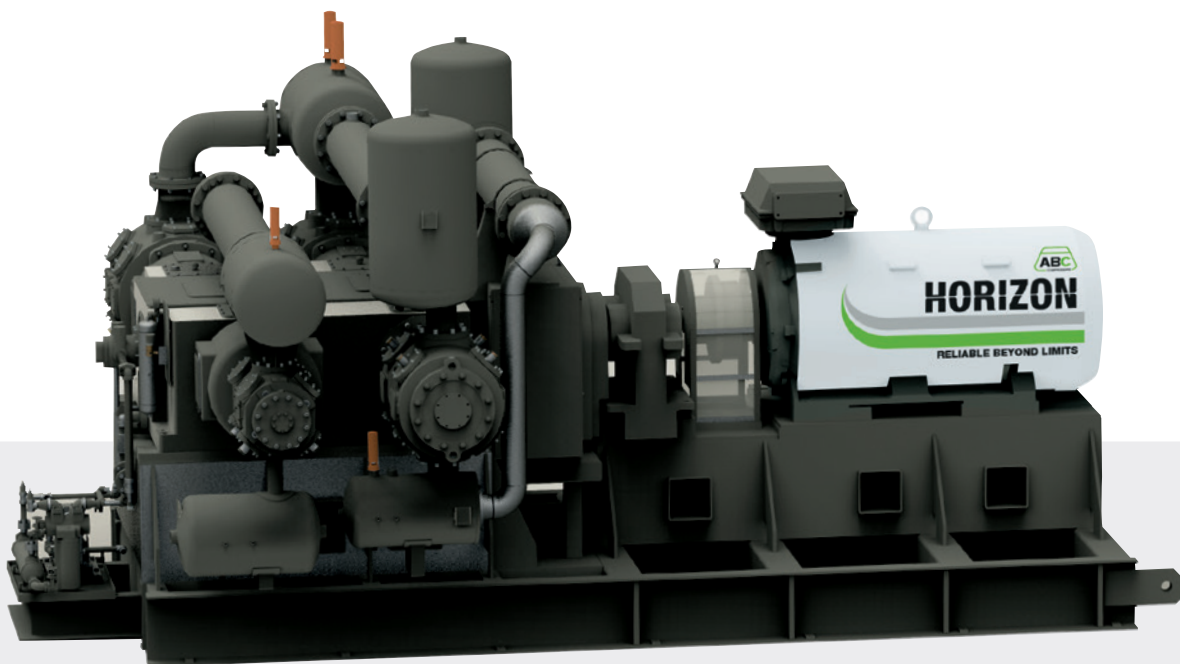
▲ HORIZON PLUS 5000 800kW
