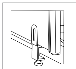
Tischadapter fasst Plattenstärken von 21 – 42 mm
