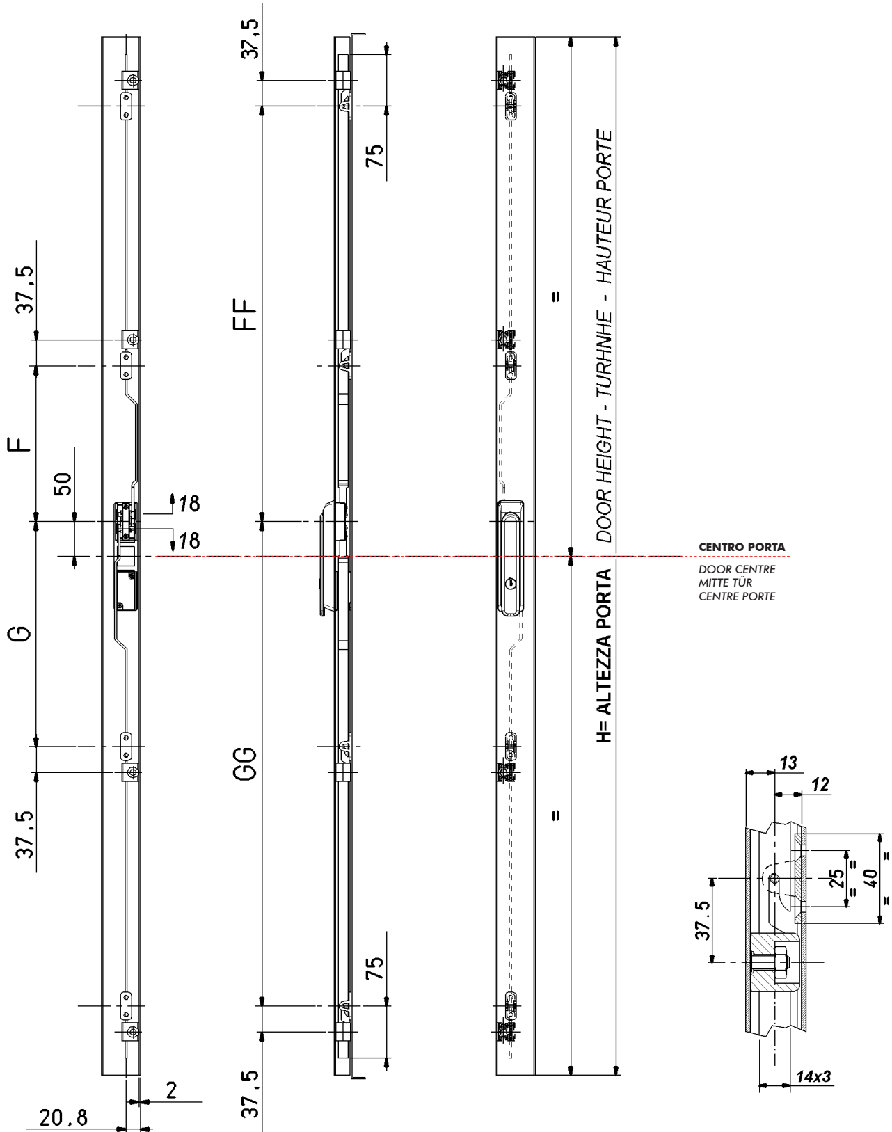
COPPIA ASTE (mm) - RODS PAIR (mm) - STANGENPAAR (mm) - PAIRE DE TRINGLES (mm)
