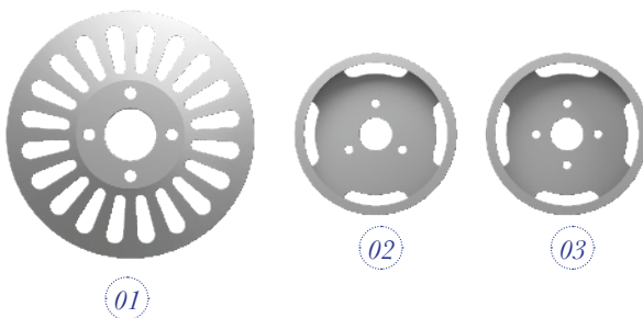
1 / Muela Ø153 2 / Muela Ø100 B64 - 3 orificios 3 / Muela Ø100 B64 - 4 orificios
