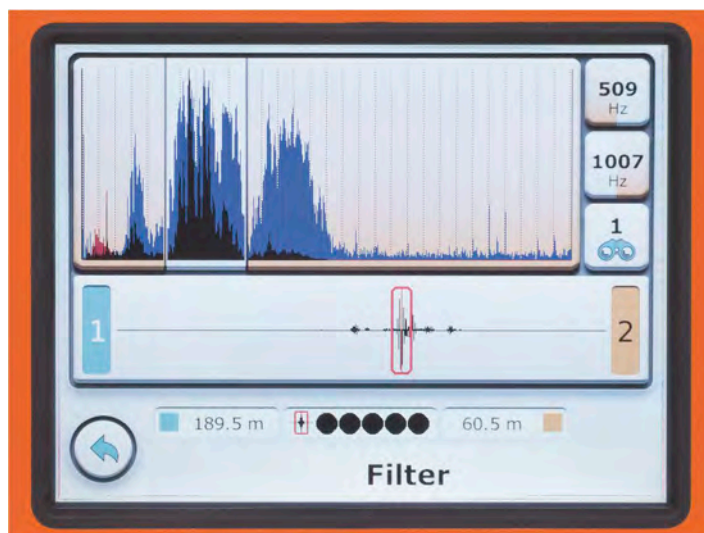
Dialogue de filtre avec des filtres automatiquement réglés
