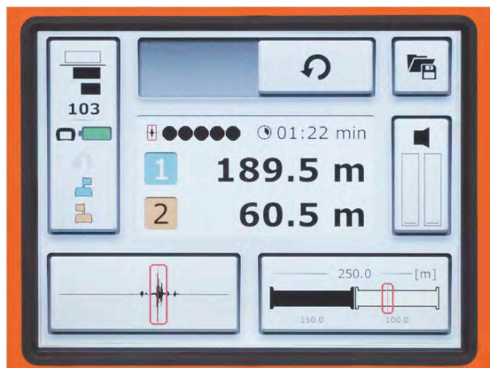
Résultat de mesure sur deux sections de canalisation
