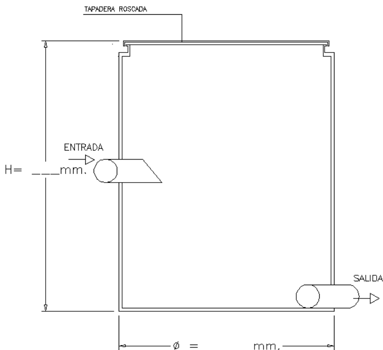
ARQUETA DE INSPECCIÓN
