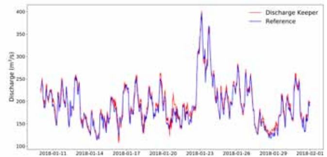
Serie cronológica del DischargeKeeper y datos de referencia
