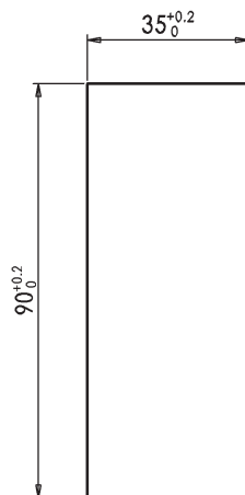
DIMENSIONI FORO DI FISSAGGIO CUT-OUT - EINBAUÖFFNUNG - PERÇAGE
